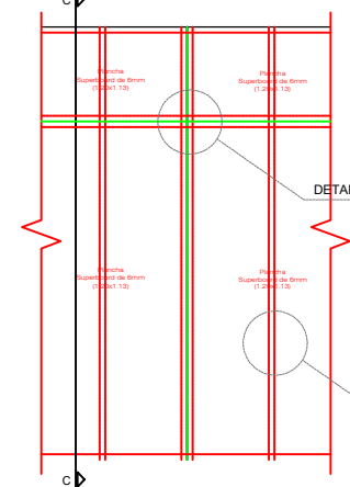
ELEVACION ESTRUCTURA TABIQUERIA ESC: 1:25
