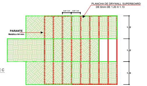
ELEVACION TABIQUERIA EXTERIOR ESC: 1:25
