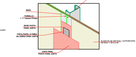
DETALLE DE JUNTA INVISIBLE
