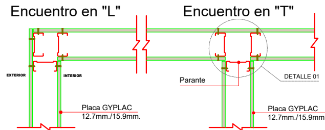
DETALLE DE ENCUENTROS
