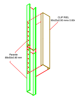
DETALLE C-C DE TRANSLAPSE EN PARANTE
